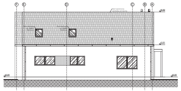
ELEWACJA BOCZNA
