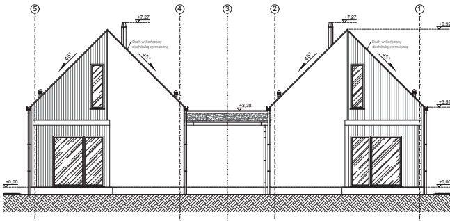
ELEWACJA TYLNA
