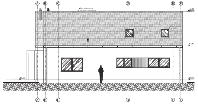
ELEWACJA BOCZNA
