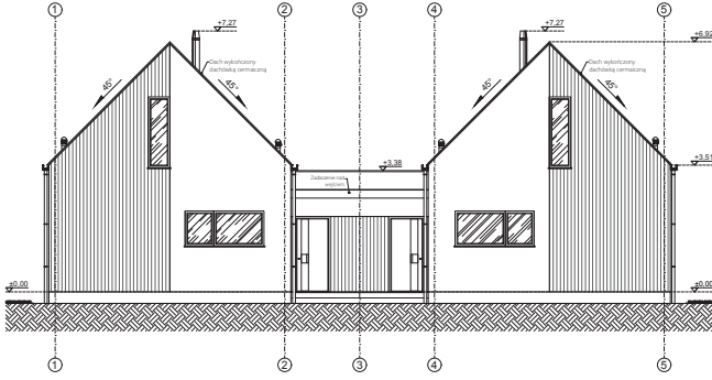
ELEWACJA FRONTOWA
